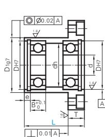
带扣环型
