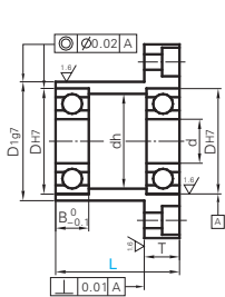
无扣环型
