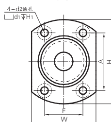
简易型
