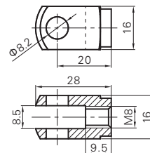
前端形状接头 (活塞杆端与气缸筒端接头)
