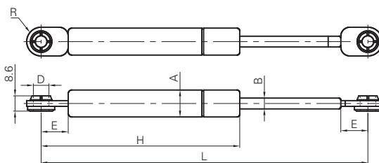
头部安装限定型 GAA
