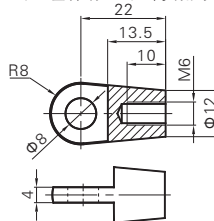
前端形状接头 (活塞杆端与气缸筒端接头)
