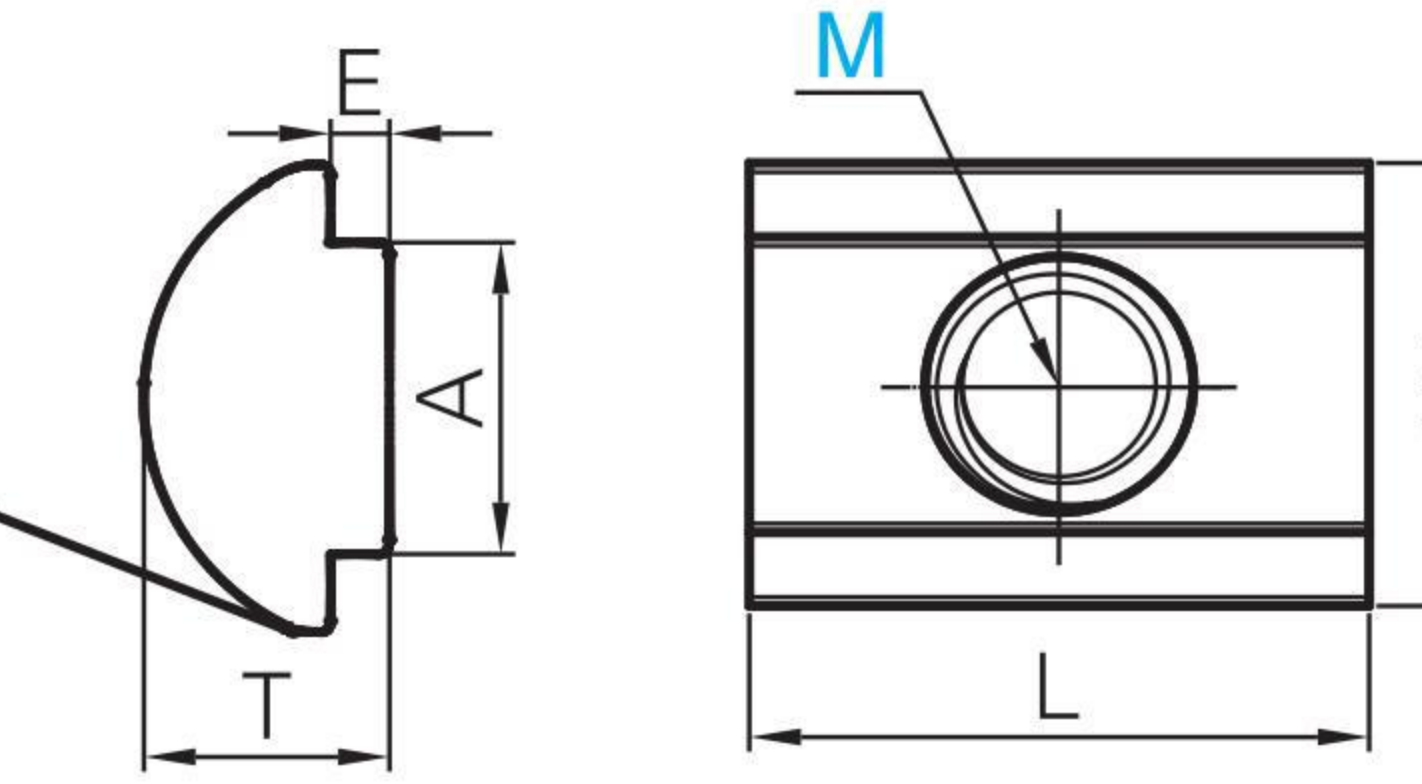
弹片螺母
