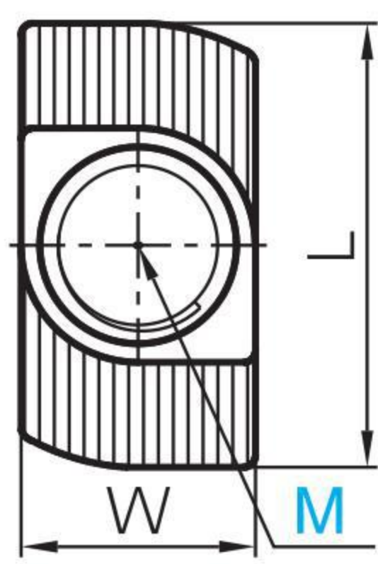
T型螺母
