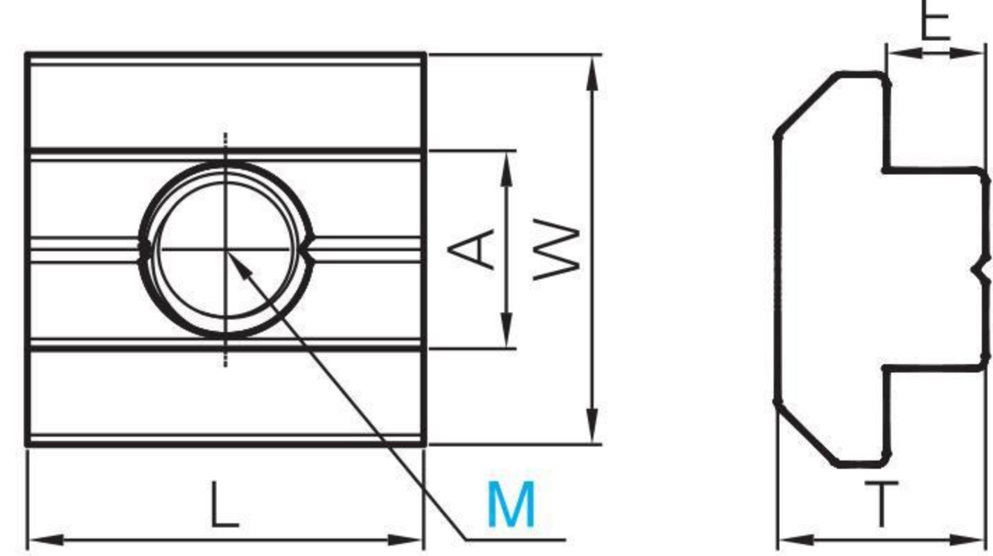
方型螺母
