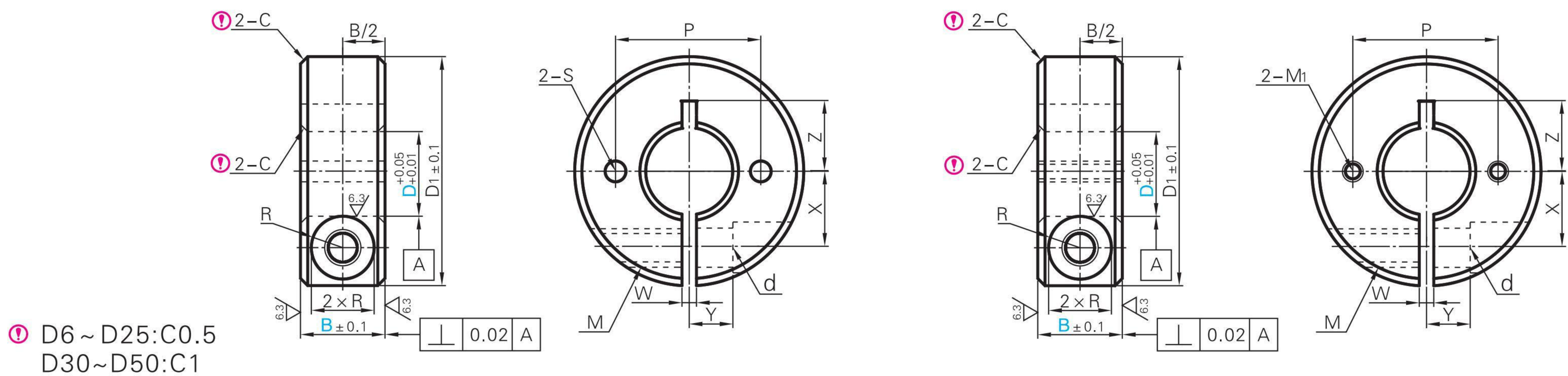
双通孔固定型
