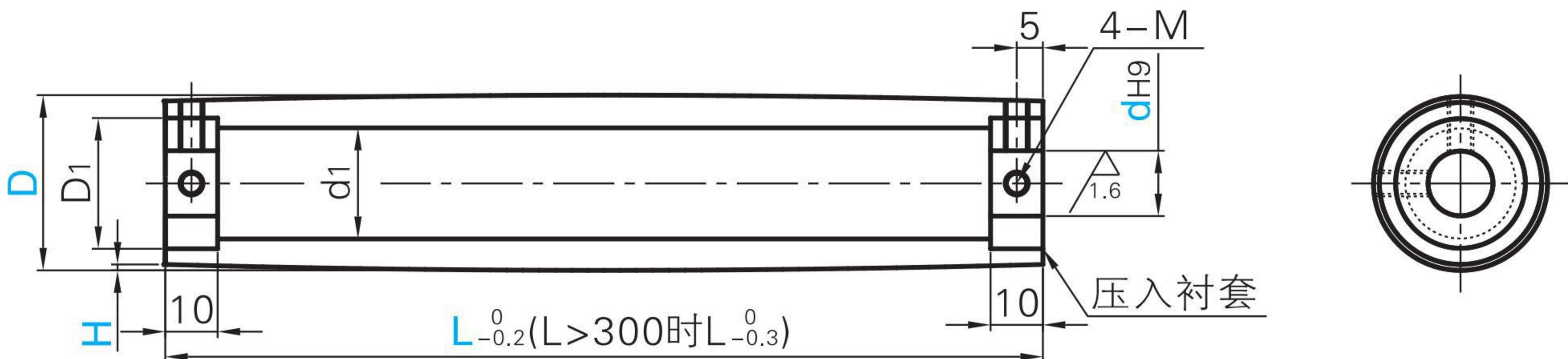
圆弧型
