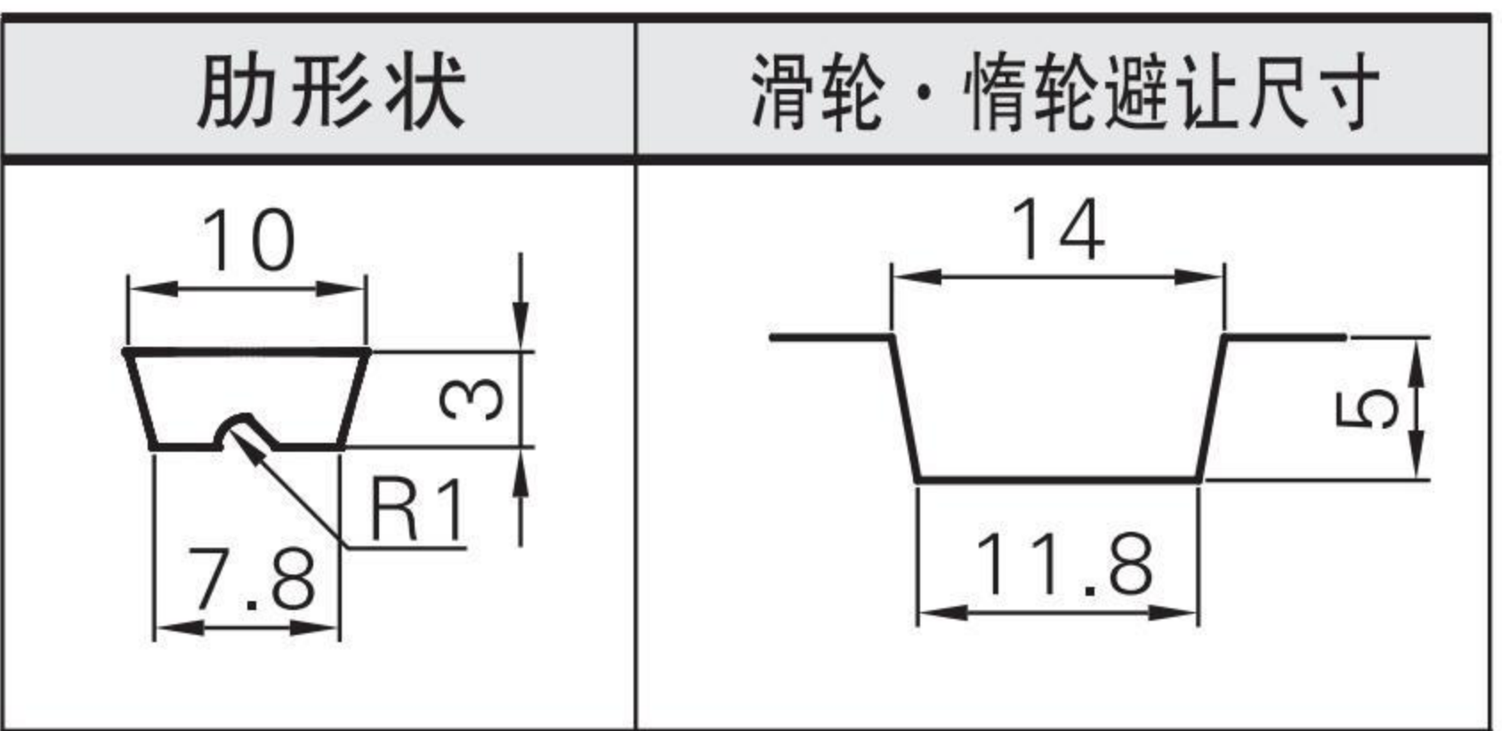
皮带的肋形状与滑轮·惰轮避让尺寸
