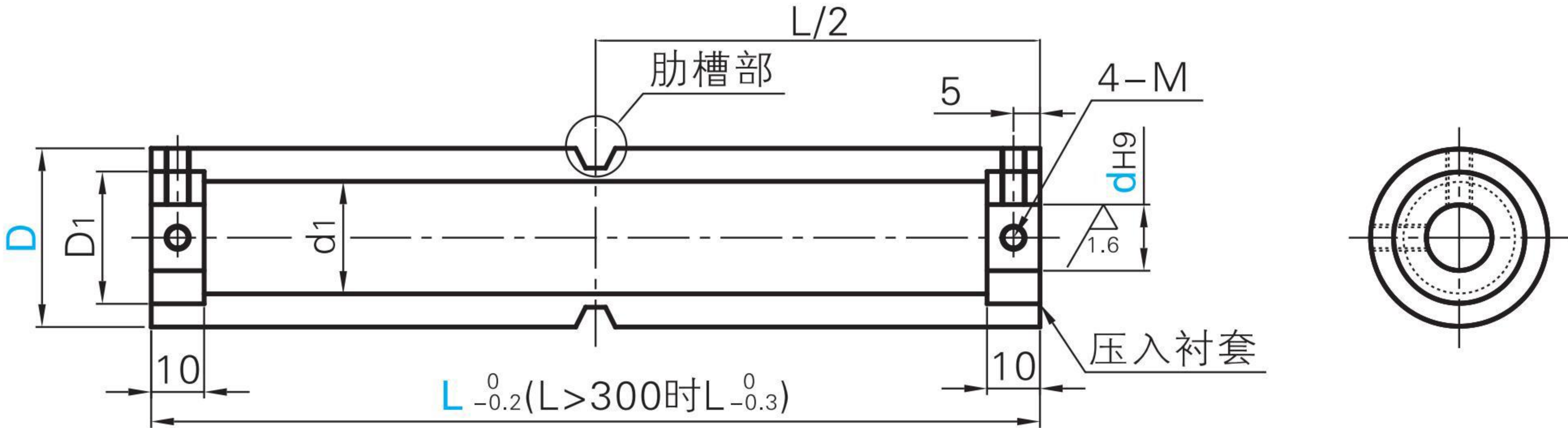
带肋槽直柱型
