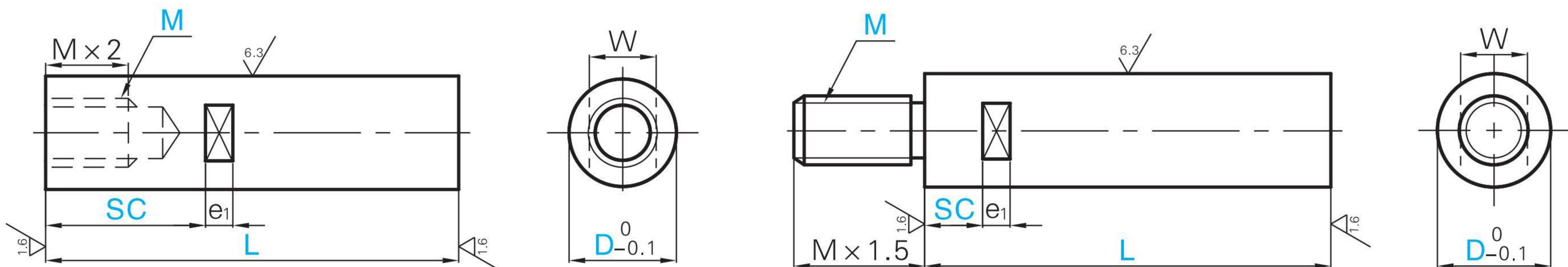
一端内螺纹
