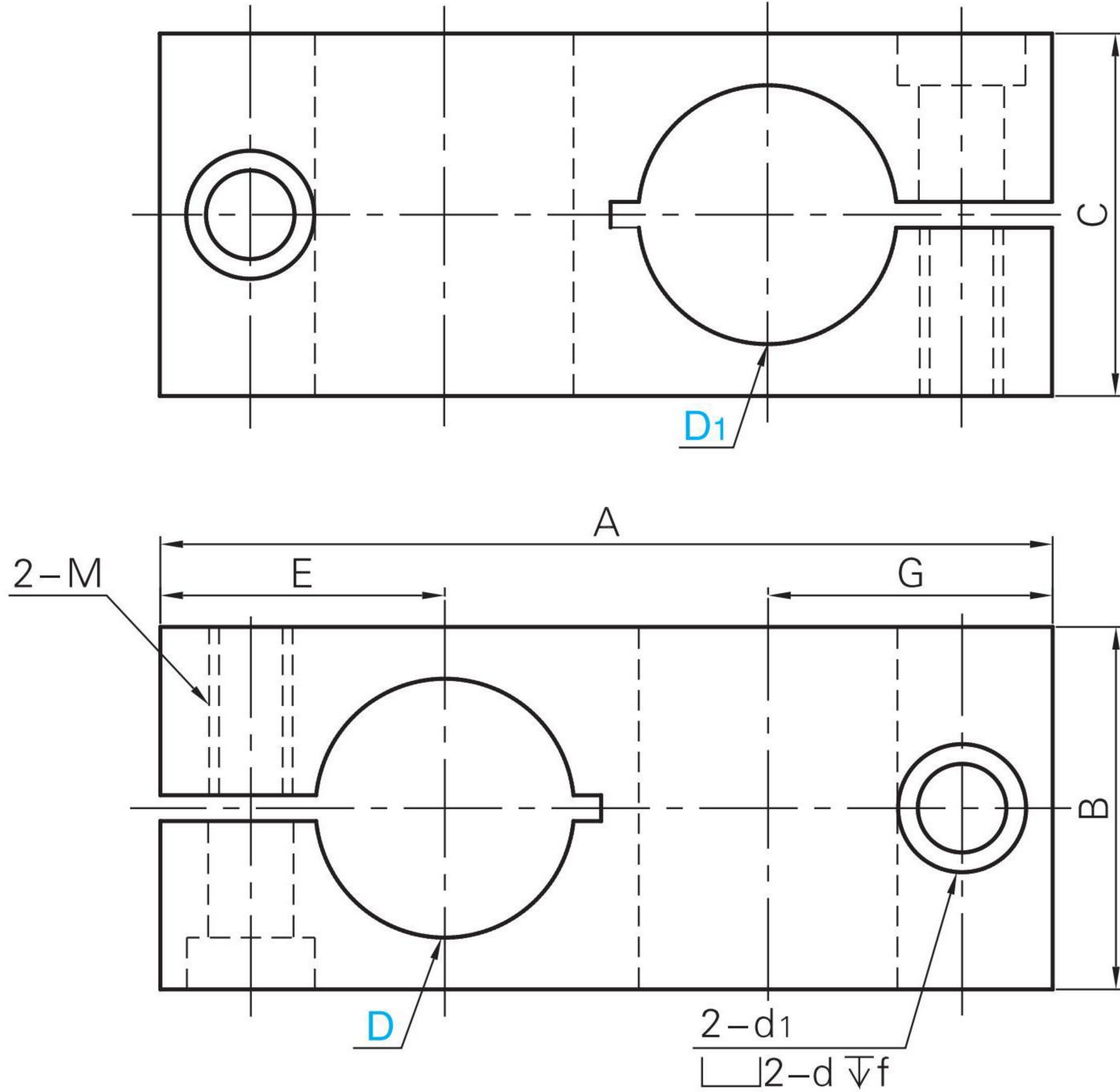
异径直交型
