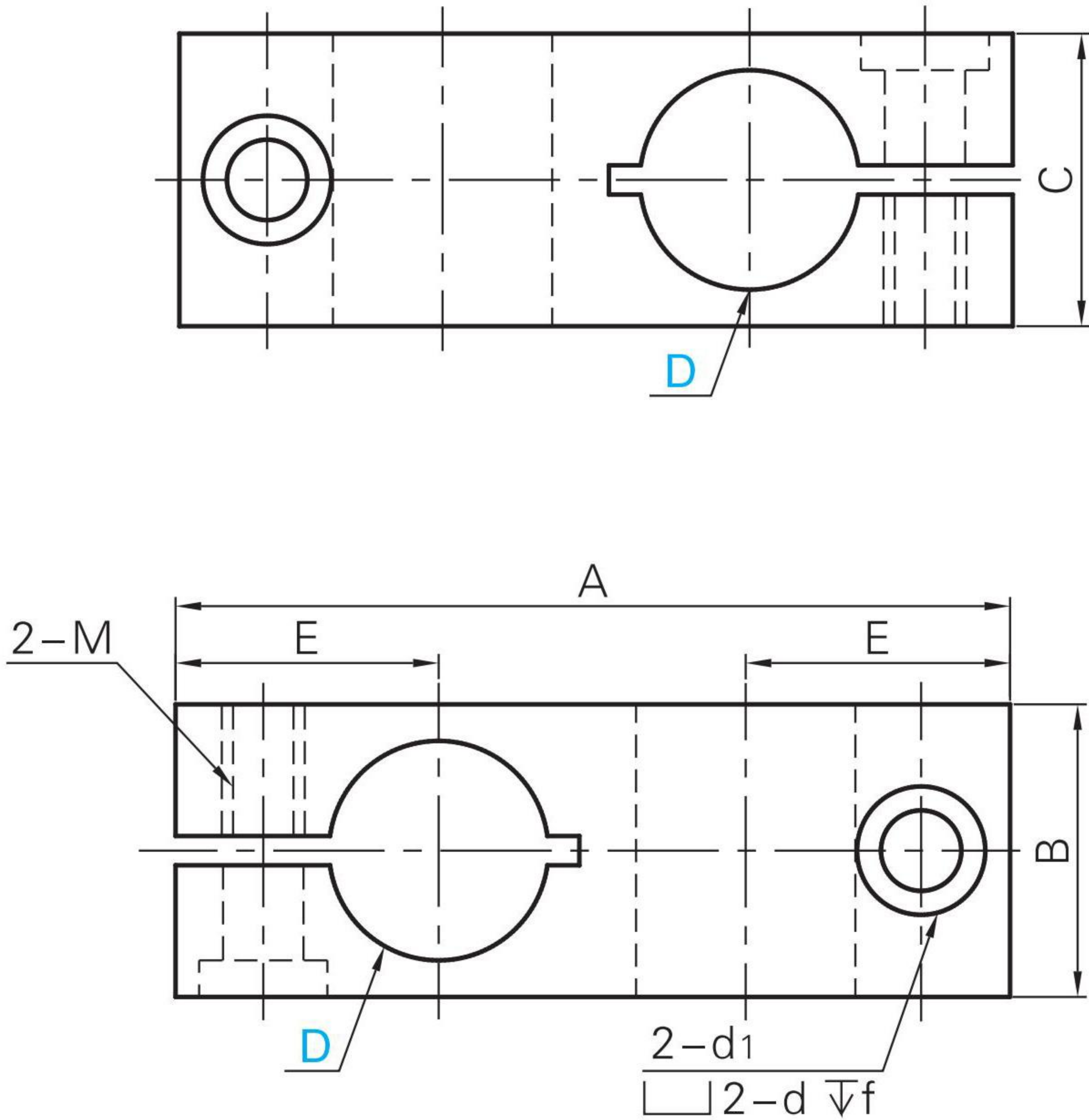
同径直交型
