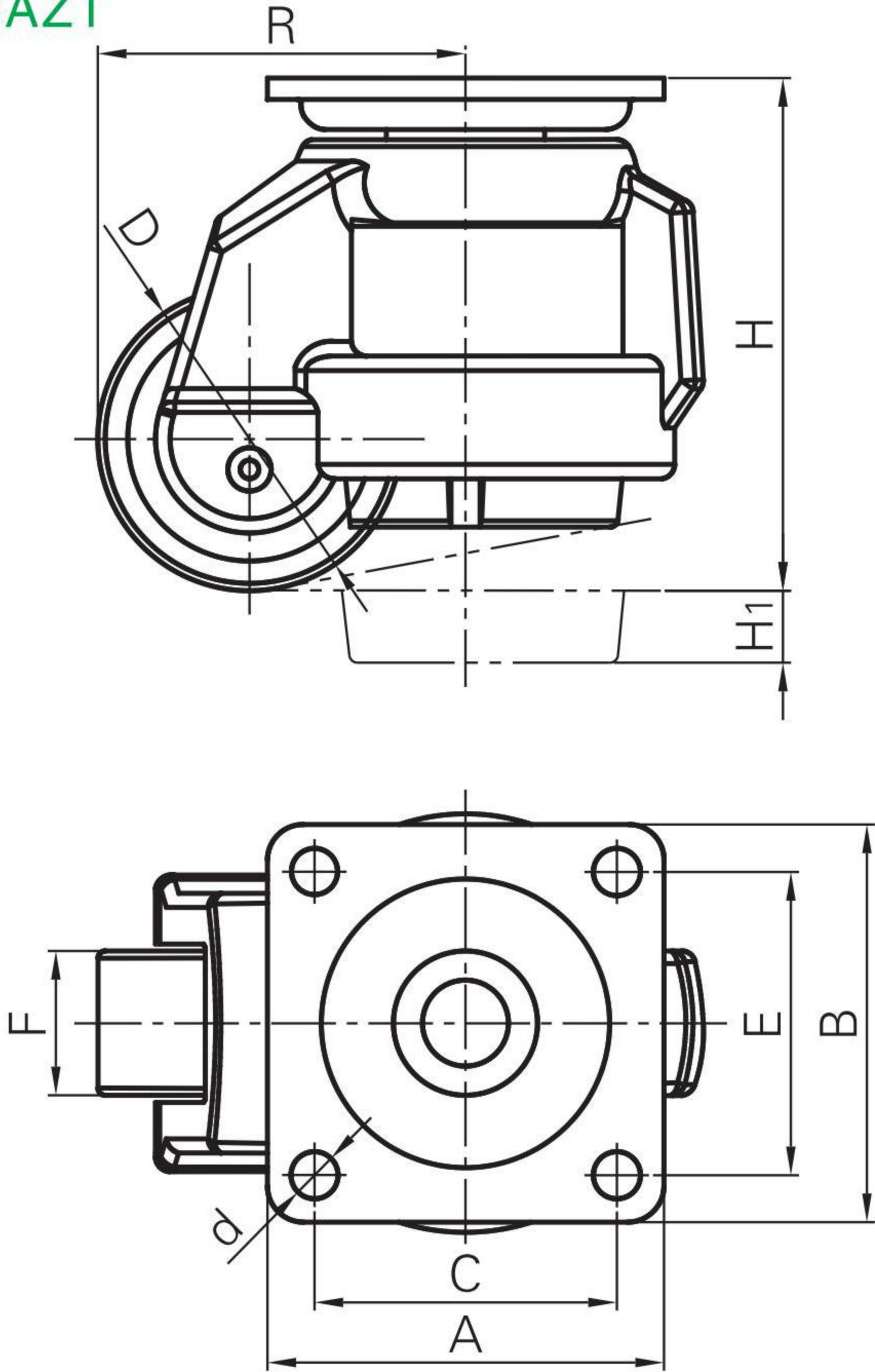
平底安装型 E-CAZT
