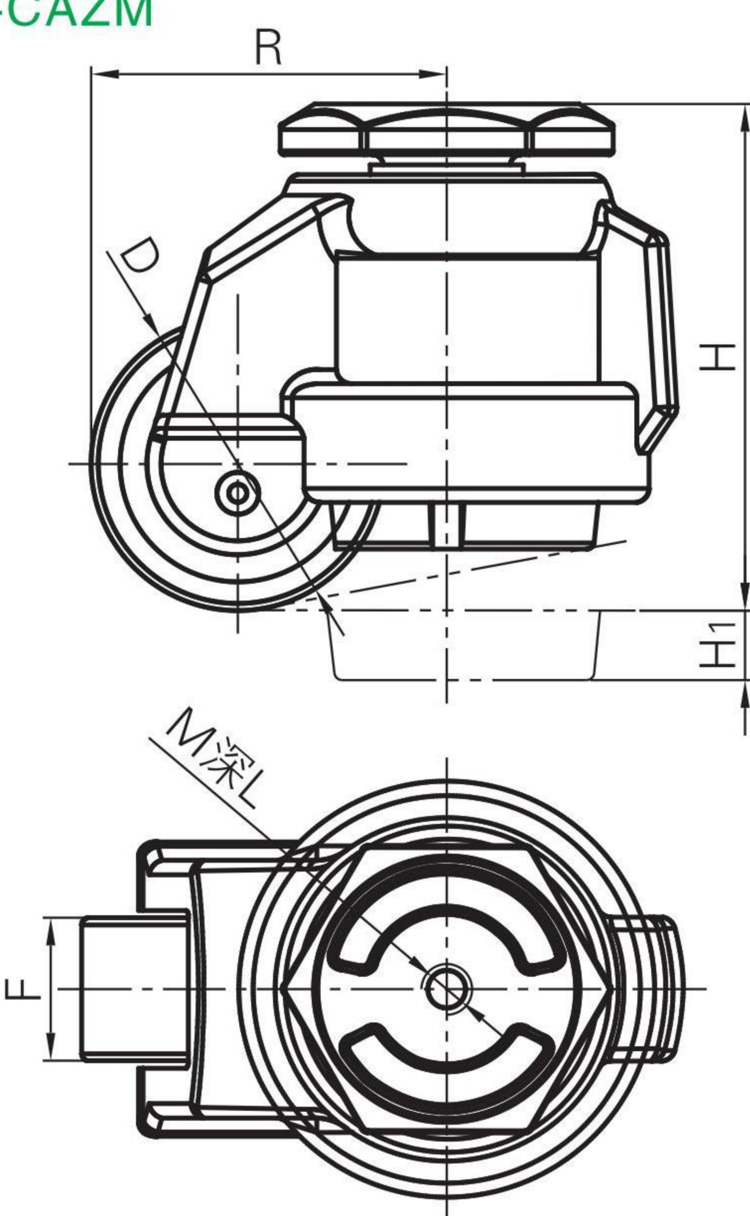
螺杆安装型 E-CAZM
