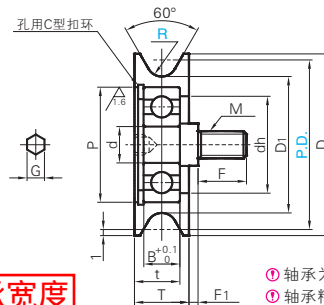
外螺纹型
