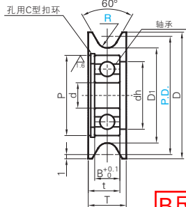
标准型
