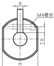
标准型
