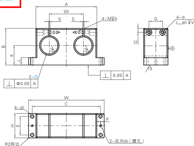
双孔型 PCFKW
