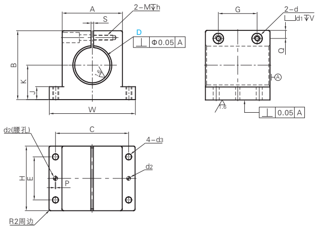
标准型 PCFK
