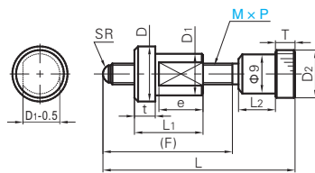
FSQK3/6 (螺牙·压花头型)
