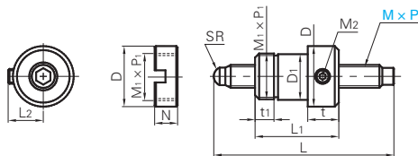
FSQR3/6/6L (螺牙·内六角头型)
