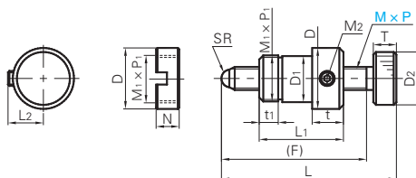
FSQR3/6/6L (螺牙·内六角头型)
