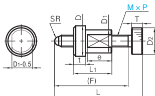
FSTR3/6/6L (圆筒·内六角头型)
