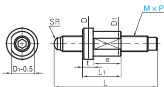
FSTR3/6/6L (圆筒·内六角头型)
