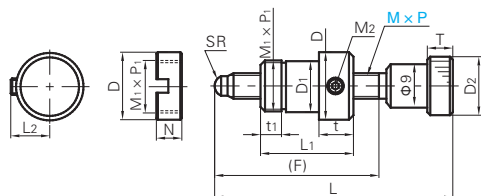
圆筒·压花头型
