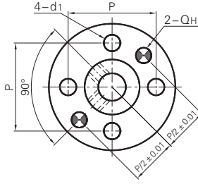
圆法兰型
