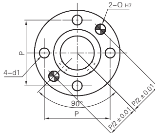
圆法兰型 No. 12~30
