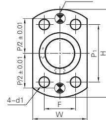
两面切割法兰型
