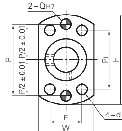
两面切割法兰型
