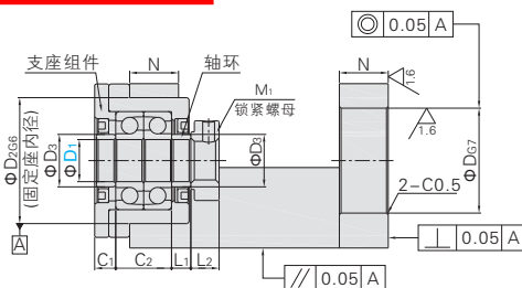
A-A向视图
