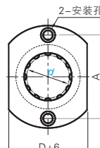
两面切割法兰型
