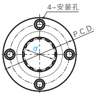
圆法兰型
