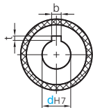
直柱型
