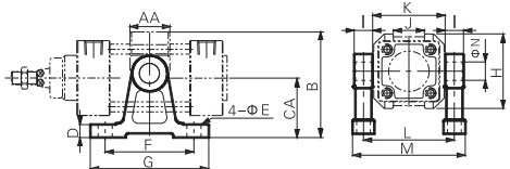
TCM1(耳轴支架)
