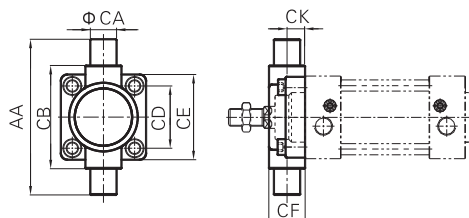
TCM1(耳轴支架)
