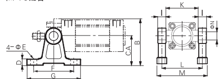
TM(耳轴支架座)
