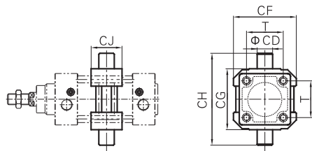
FTC(前盖耳轴支架)
