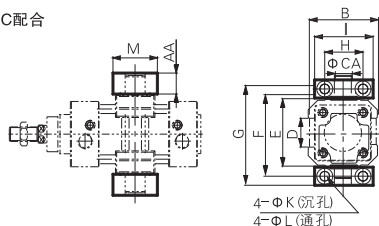
TM(耳轴支架座)
