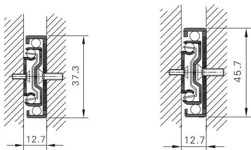
安装示意图
